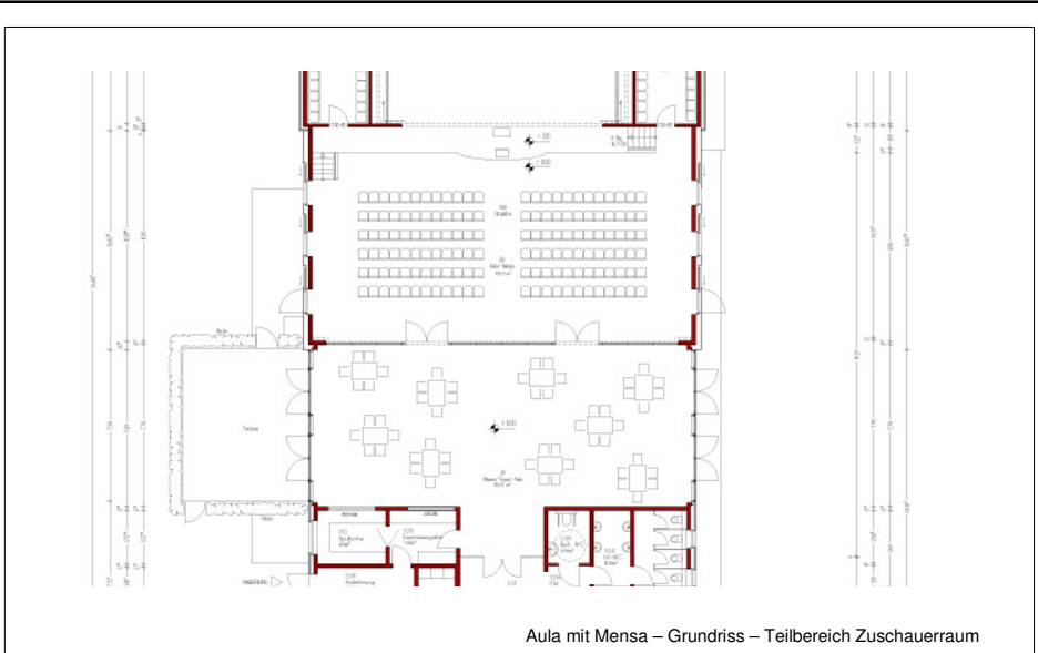
Aula mit Mensa – Grundriss – Teilbereich Zuschauerraum
