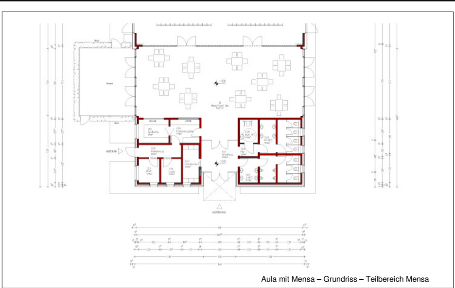
Aula mit Mensa – Grundriss – Teilbereich Mensa
