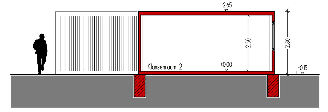
Schnitt A-A
