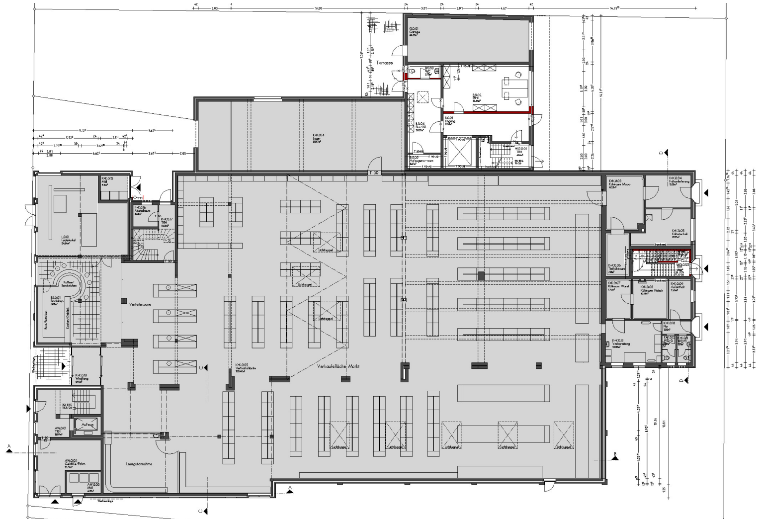
Erdgeschoss gesamt
