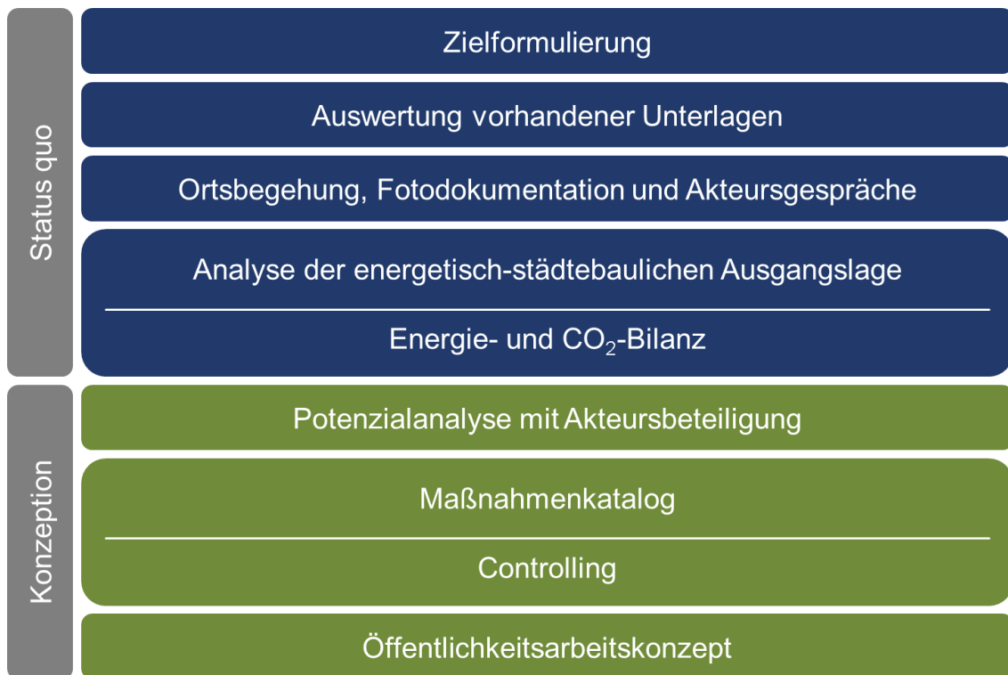
Abbildung 1-9: Aufbau des integrierten energetischen Quartierskonzeptes (Eigene Darstellung)
