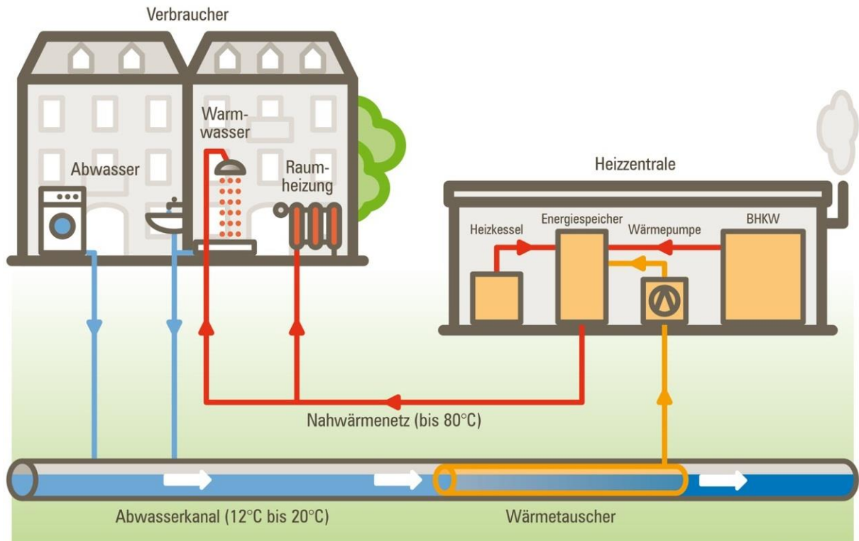
Abbildung 3-18: Wirkschema der Abwasserwärmenutzung 25
