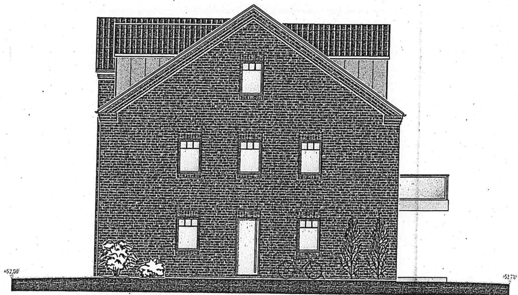
ANSICHT NORDEN
