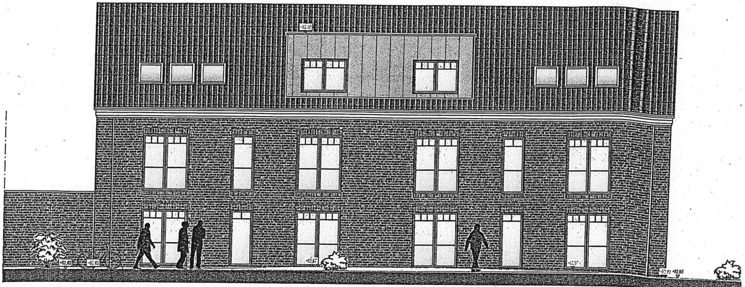
ANSICHT WESTEN
