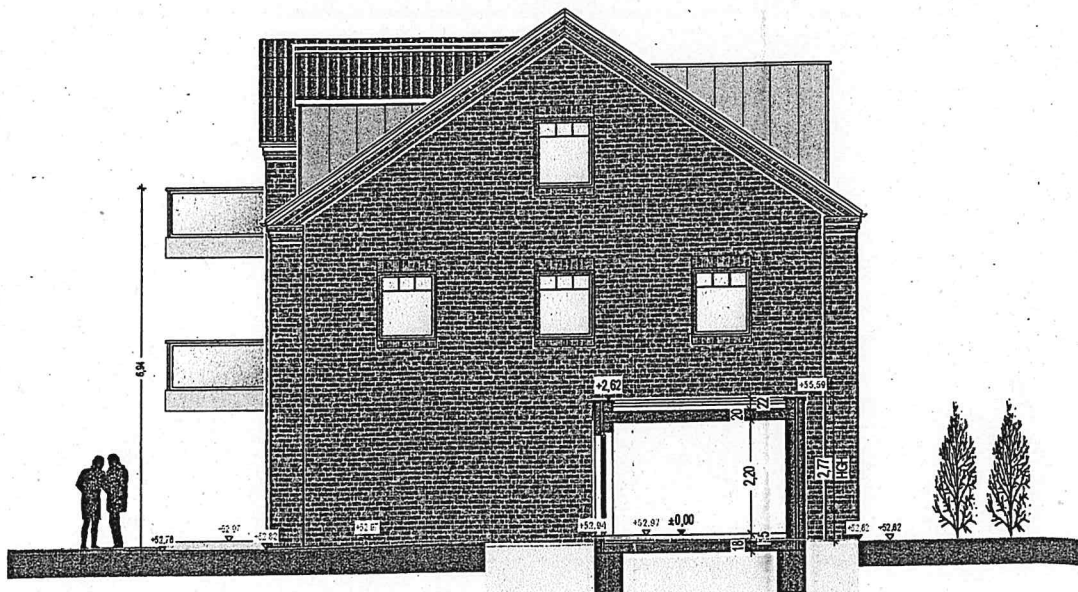
ANSICHT NORDEN
