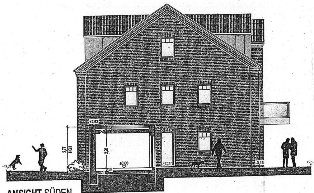
ANSICHT SÜDEN.
